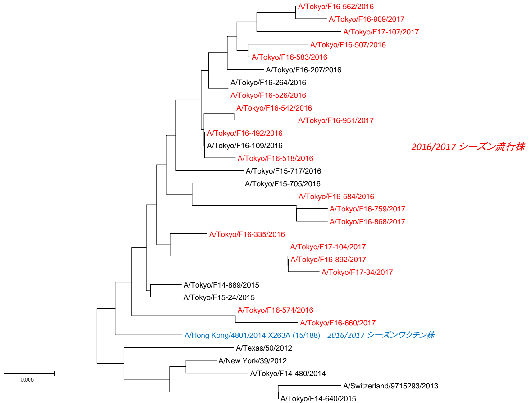
図2. 東京都におけるAH3亜型インフルエンザウイルスのHA遺伝子系統樹
