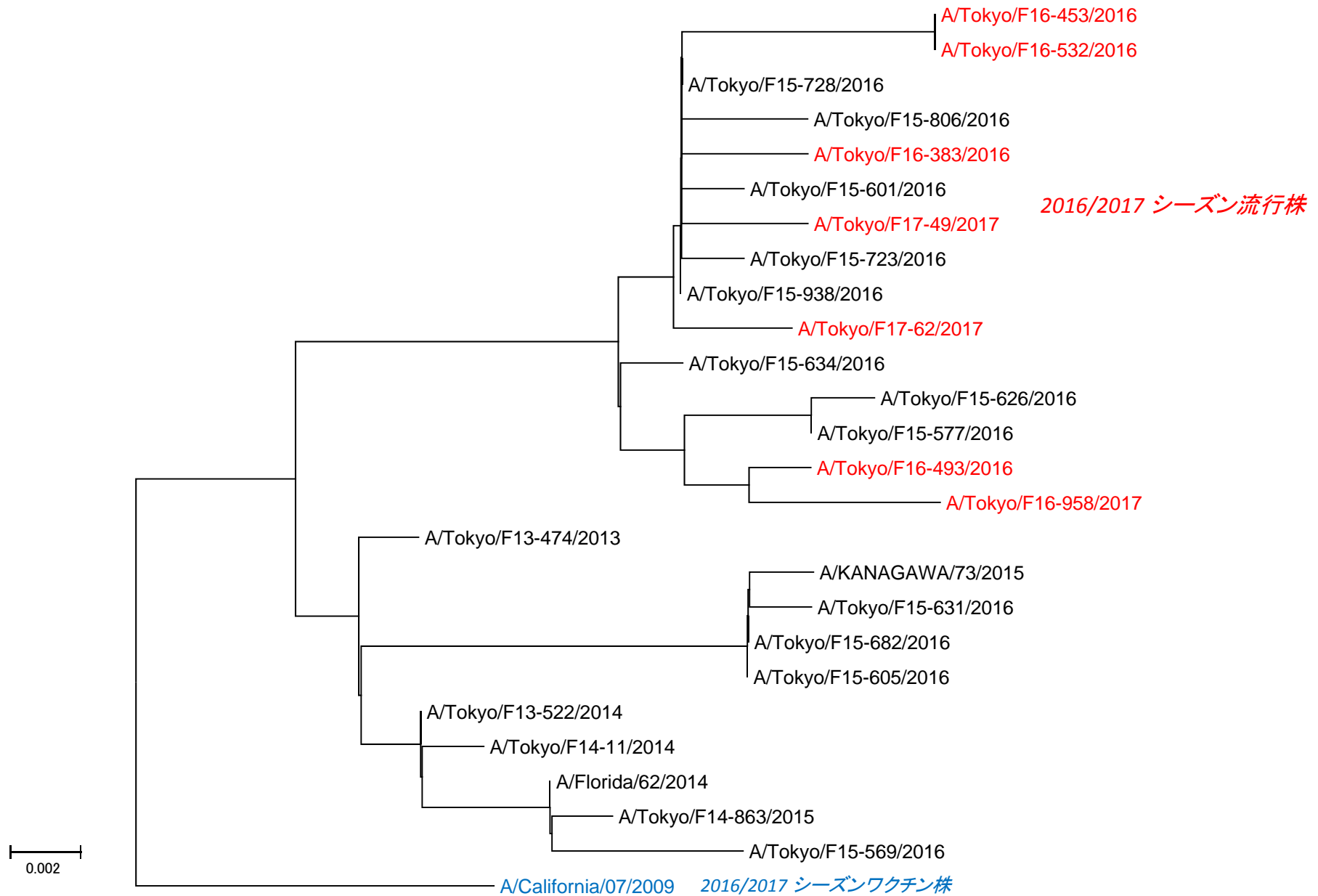
図1. 東京都におけるAH1pdm09インフルエンザウイルスのHA遺伝子系統樹
